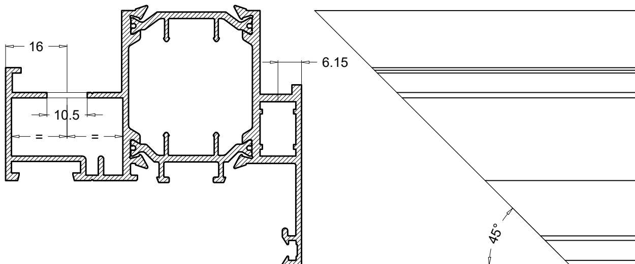
SECTION A-A
