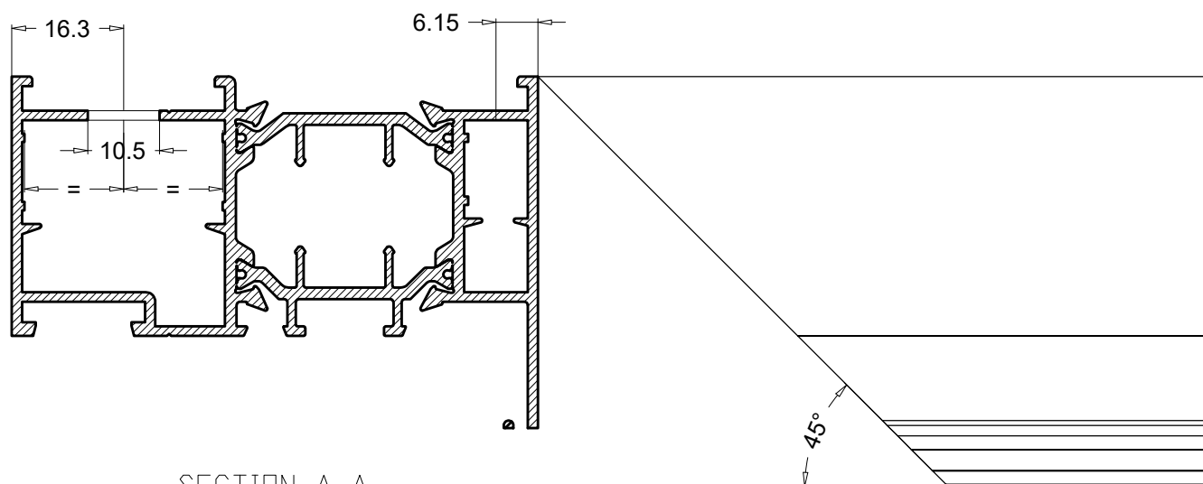
SECTION A-A
