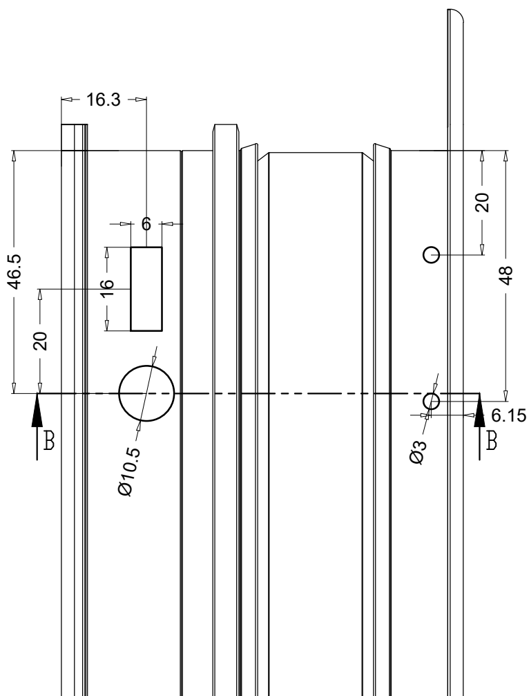
SECTION A-A
